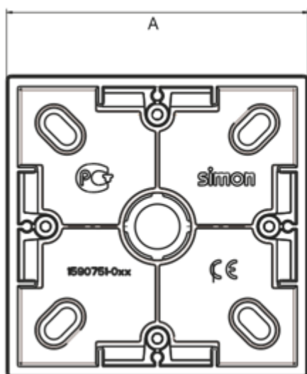
Рисунок 1. КОРОБКА ДЛЯ НАРУЖНЕГО МОНТАЖА
